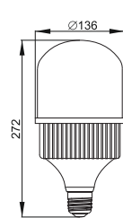
Рисунок 35 – Лампа LED-HP, 80 Вт, 100 Вт, цоколь E40
