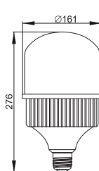
Рисунок 34 – Лампа LED-HP, 65 Вт, цоколь E40
