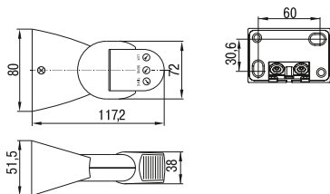
Рисунок 8 – ДД-МВ501
