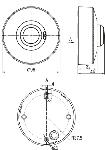
Рисунок 4 – ДД-МВ101
