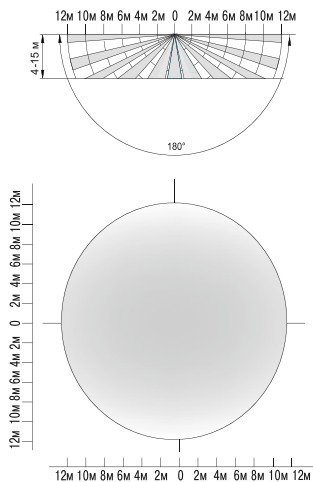
Рисунок 3 – ДД-МВ601
