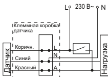
Рисунок 7 – Схема режима с постоянным включением нагрузки
