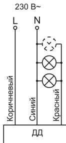
Рисунок 5 – Схема подключения датчиков ДД 024 и ДД 024В
