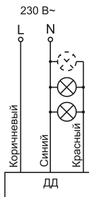
Рисунок 5 – Схема подключения датчиков ДД 024 и ДД 024В
