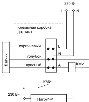
Рисунок 28 – Схема подключения датчика с контактором КМИ
