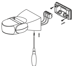
Рисунок 16 – Монтаж ДД 013
