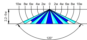
Рисунок 1 – ДД 013, ДД 015, ДД 016
