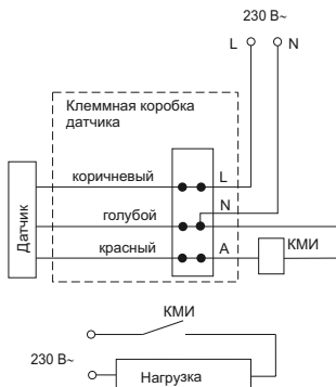
Рисунок 28 – Схема подключения датчика с контактором КМИ
