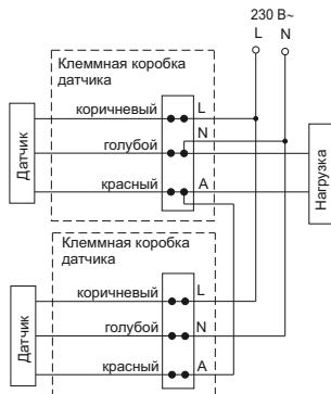
Рисунок 26 – Схема параллельного подключения датчиков
