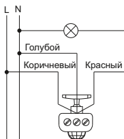
Рисунок 25 – Схема подключения датчика типа ДД 046
