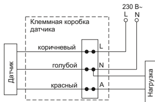
Рисунок 23 – Схема подключения датчиков типов: ДД 022, ДД 023
