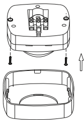
Рисунок 18 – Монтаж ДД 022, ДД 023
