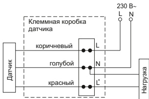
Рисунок 22 – Схема подключения датчиков типов: ДД 013, ДД 015, ДД 016
