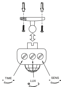
Рисунок 21 – Монтаж ДД 046
