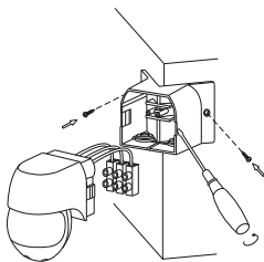
Рисунок 17 – Монтаж ДД 015, ДД 016
