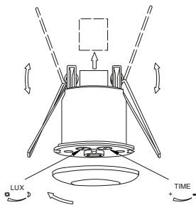
Рисунок 20 – Монтаж ДД 043
